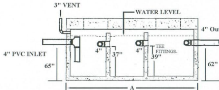
SECTION:ELEVATION
